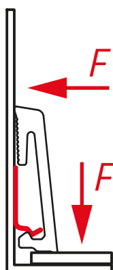
Opcja 2. (do gotowej podłogi) Plastikowy klips na wkrętę
